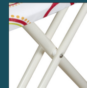
Estructura de gran estabilidad: 1 tubo \varnothing 30 mm + 2 \varnothing 22 mm.
